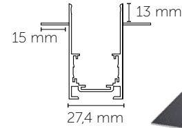
Siva Altı/Trimless Alüminyum Ray Recessed/Trimless Aluminium Track
